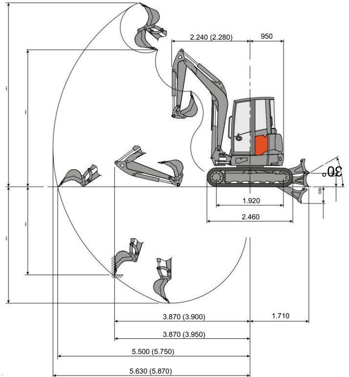
Brazo de excavación estándar L=1.500 (brazo de excavación opcional L=1.750)
