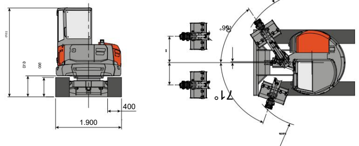
Brazo de excavación estándar L=1.500 (brazo de excavación opcional L=1.750)
