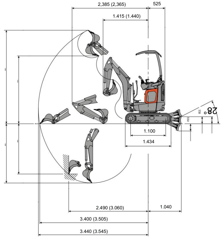
Brazo de excavación estándar L=900 (brazo de excavación opcional L=1.020)
