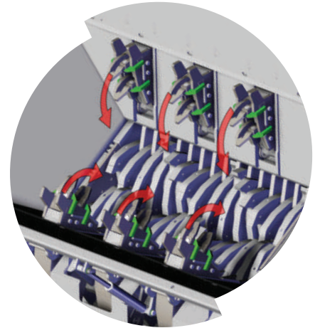
EMPUJADORES HIDRÁULICOS
